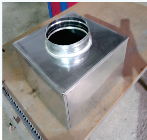
Hộp gió cho cửa gió vuông
