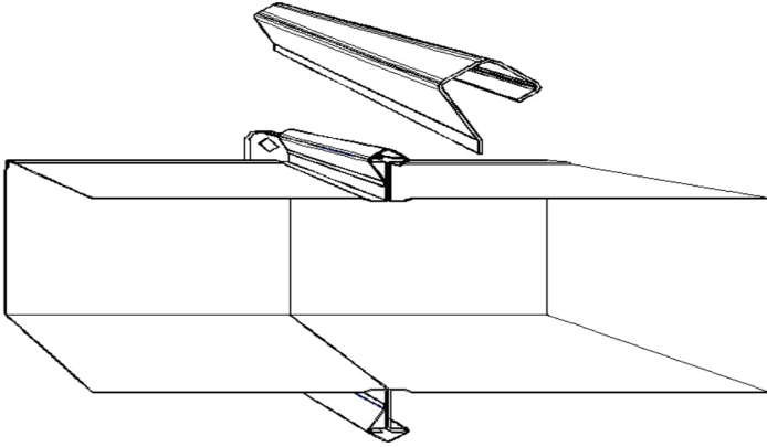
Loại 1 Ống gió vuông kẹp bích TDC
