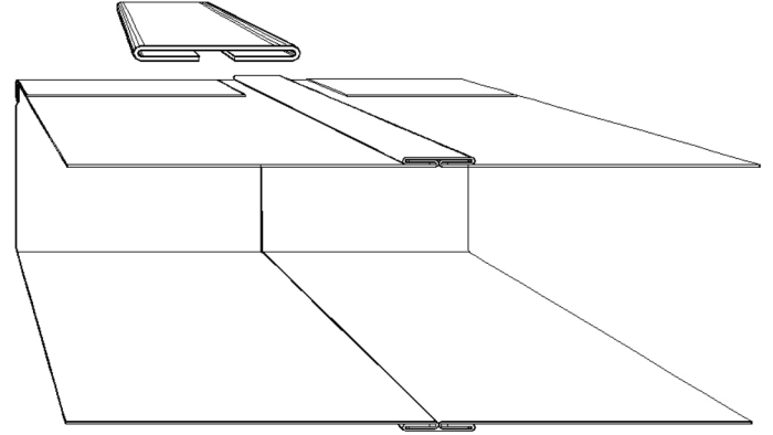
Loại 2 Ống gió vuông nẹp C
